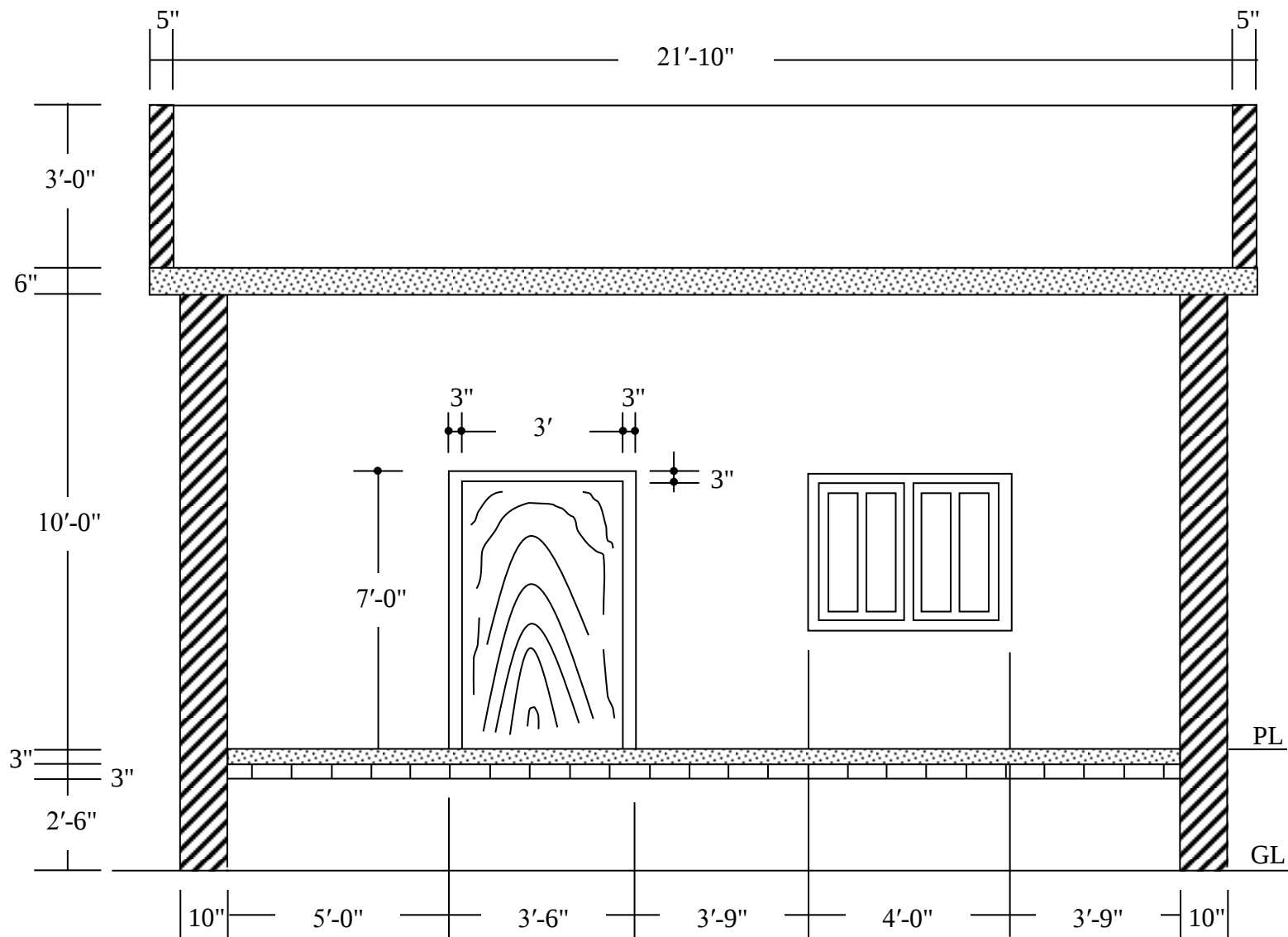
Section A-A
